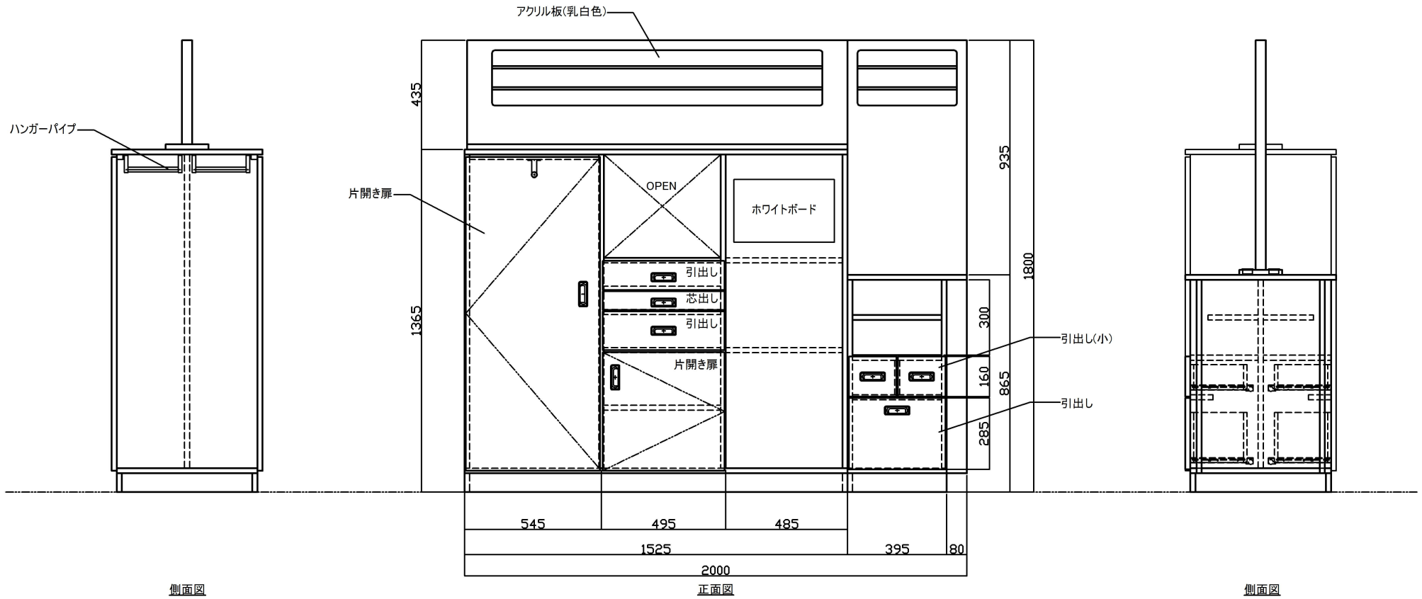
側面図
